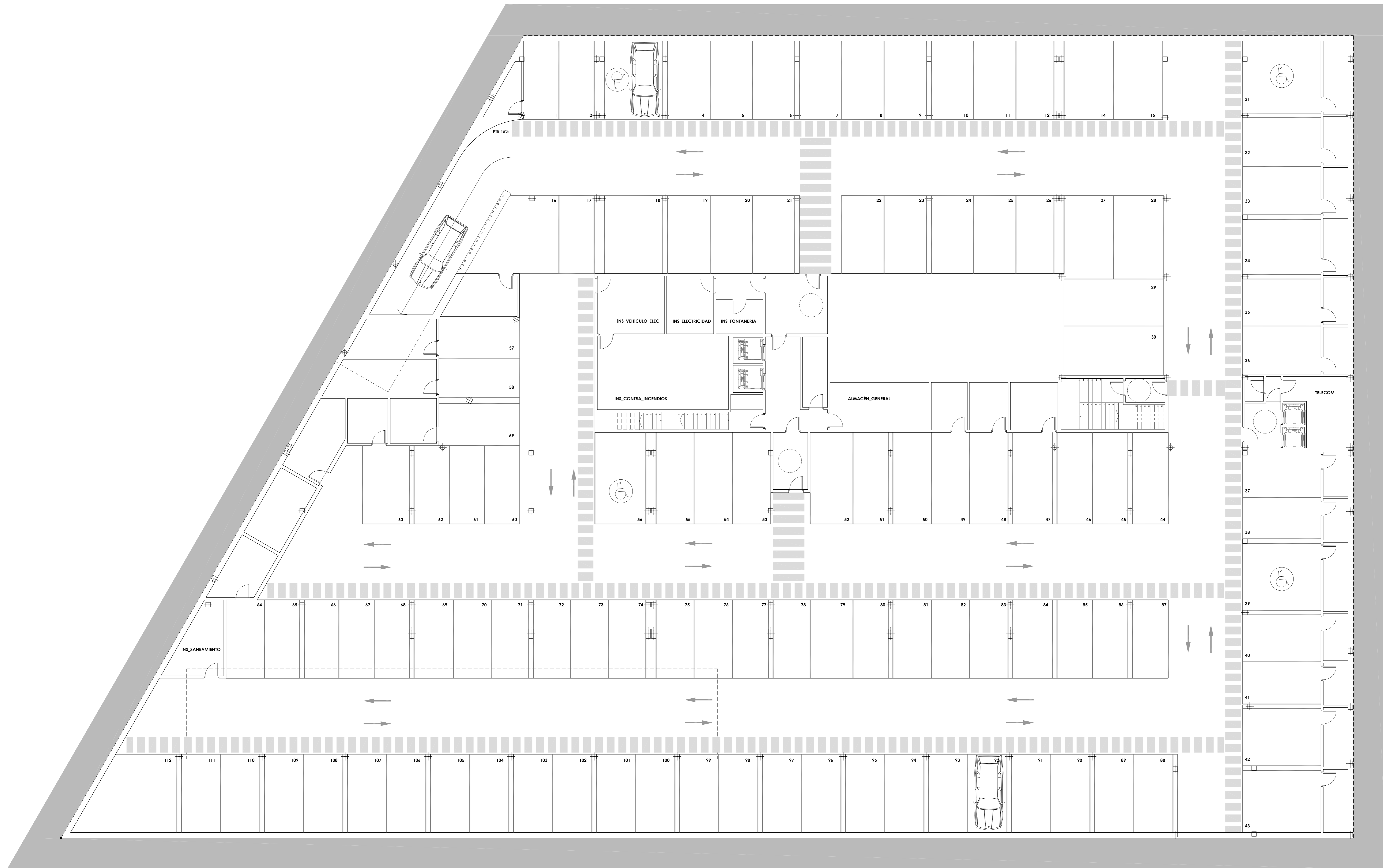
PLANTA DE SÓTANO ESCALA 1/100
